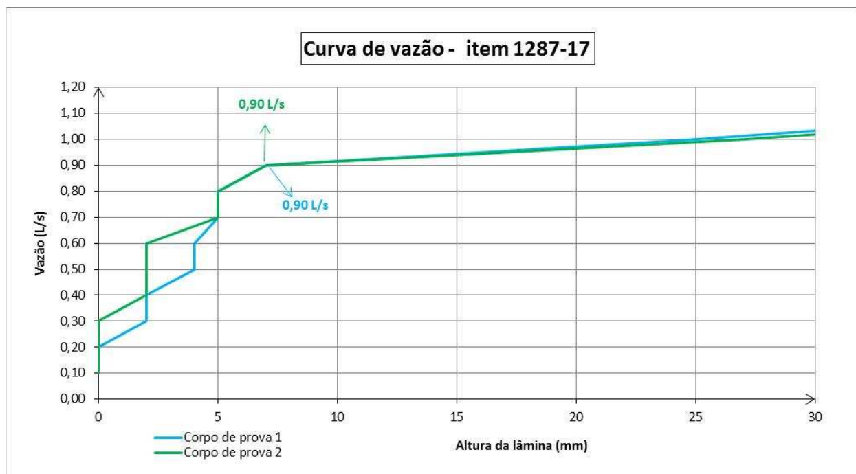
Figura 1 – Curva de vazão – item 1287-17
