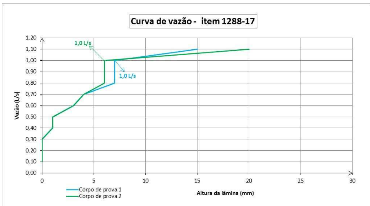
Figura 1 – Curva de vazão – item 1288-17
