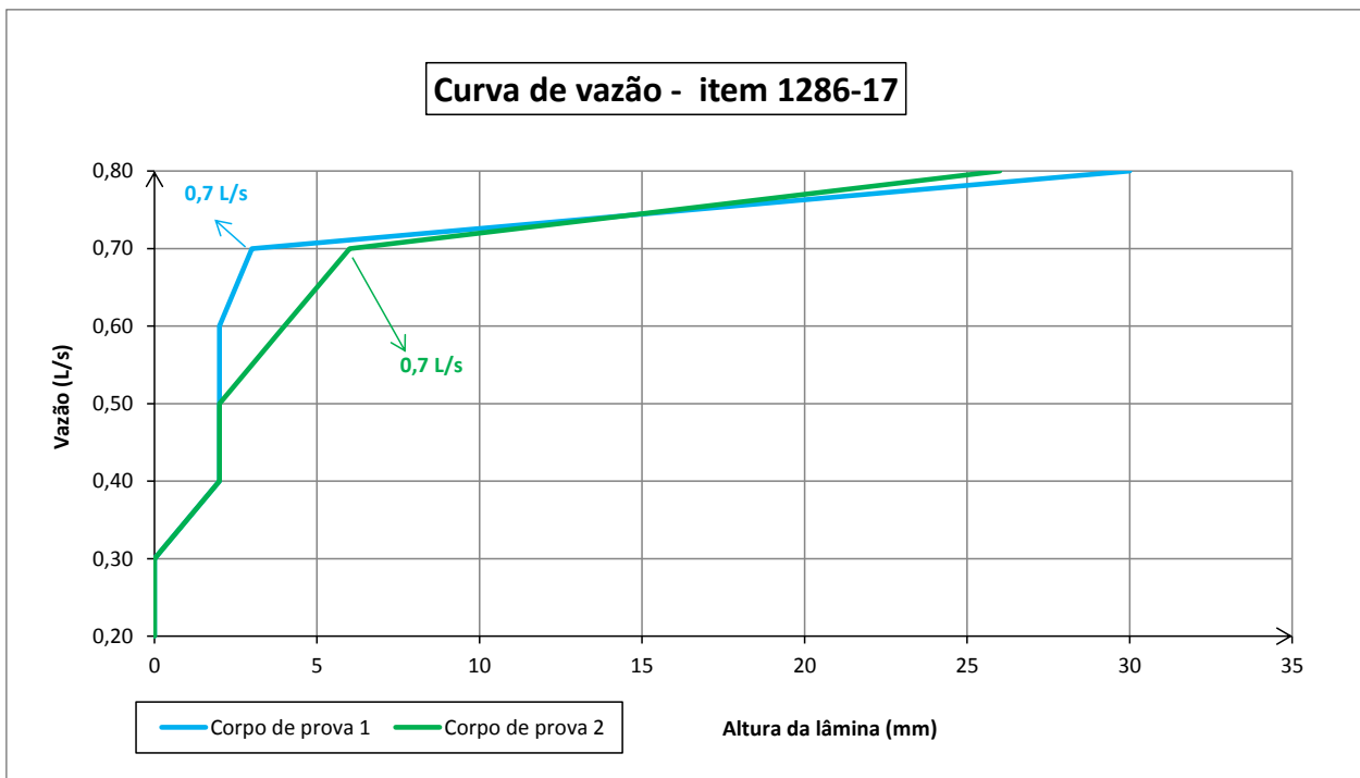
Figura 1 – Curva de vazão – item 1286-17
